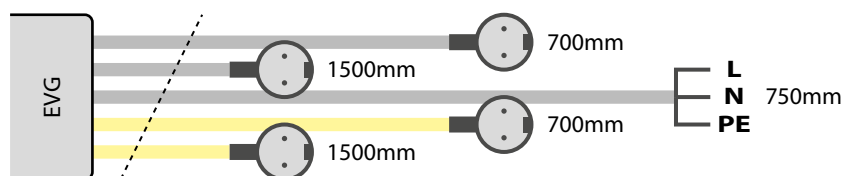
Kabellängen (2-flammig)
