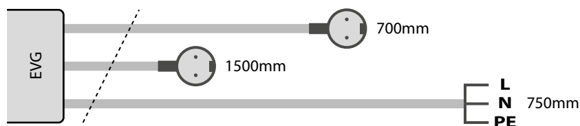
Kabellängen (1-flammig)
